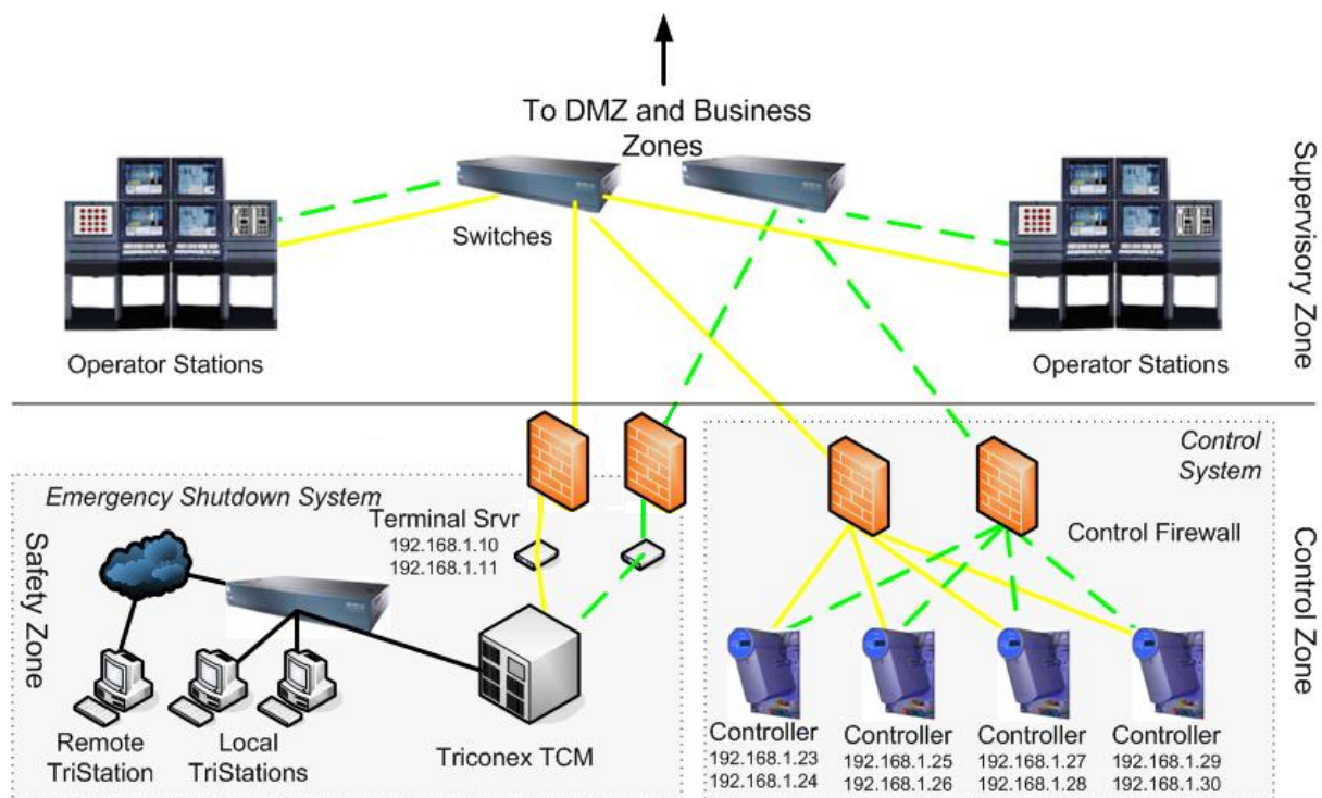
Figura 3. Arquitetura ilustrada da zona S1 protegida.
