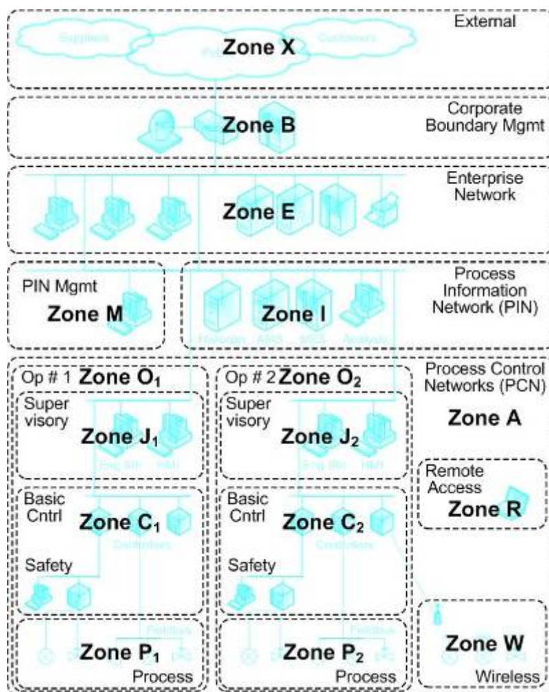
Figura 2. Rede de automação da refinaria dividida em zonas de segurança.
