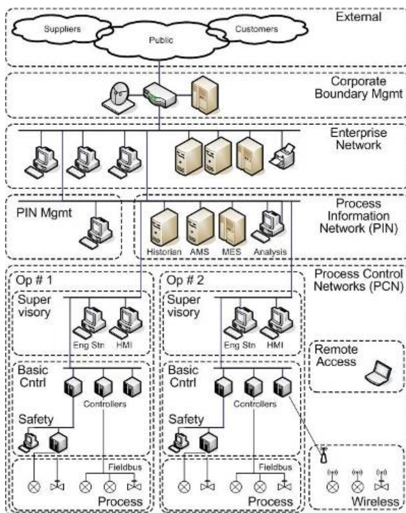
Figura 1. Topologia da rede de automação da refinaria.
