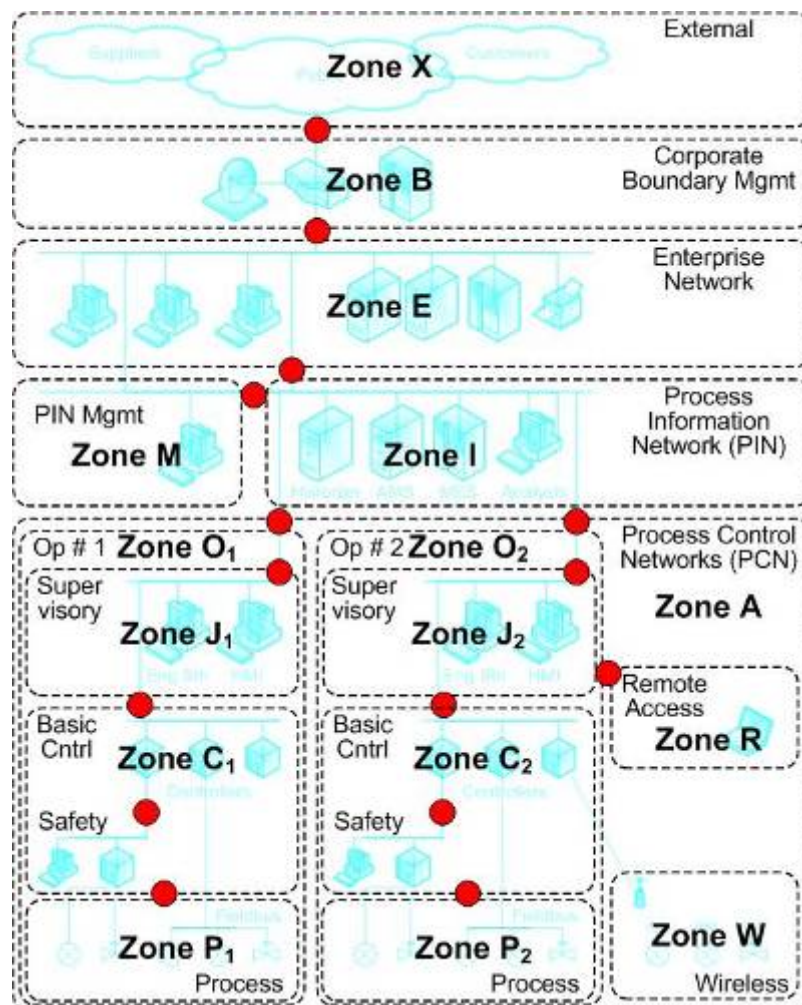
Figura 3. Conduítes apresentados entre as zonas de segurança.
